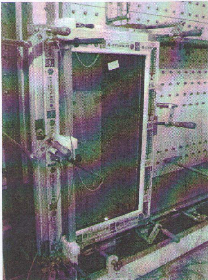
Fereastra în stand, echipată cu senzorii de deplasare
