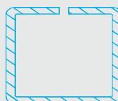
A3052 // 25x35x2
